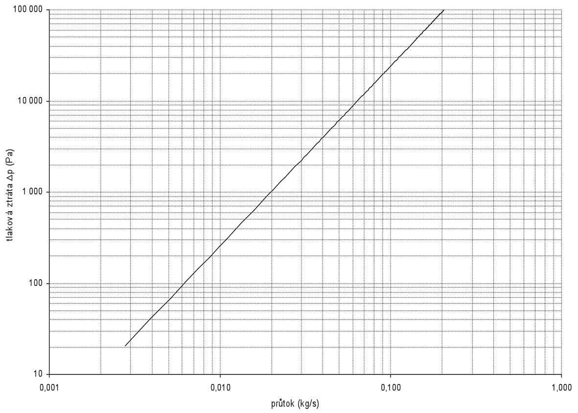
tlaková ztráta ventilového spodku k termostat. hlavici 1/2" přímý
