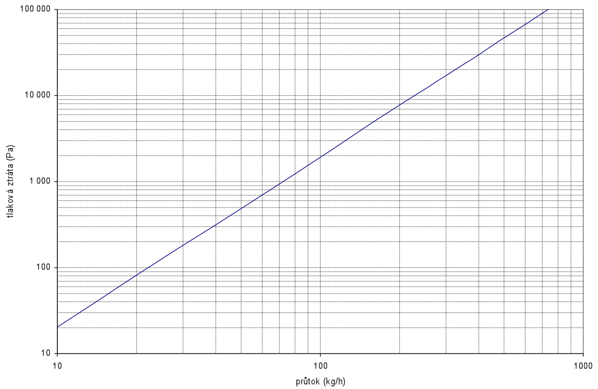
tlaková ztráta ventilového spodku k termostatické hlavici 1/2" přímého
