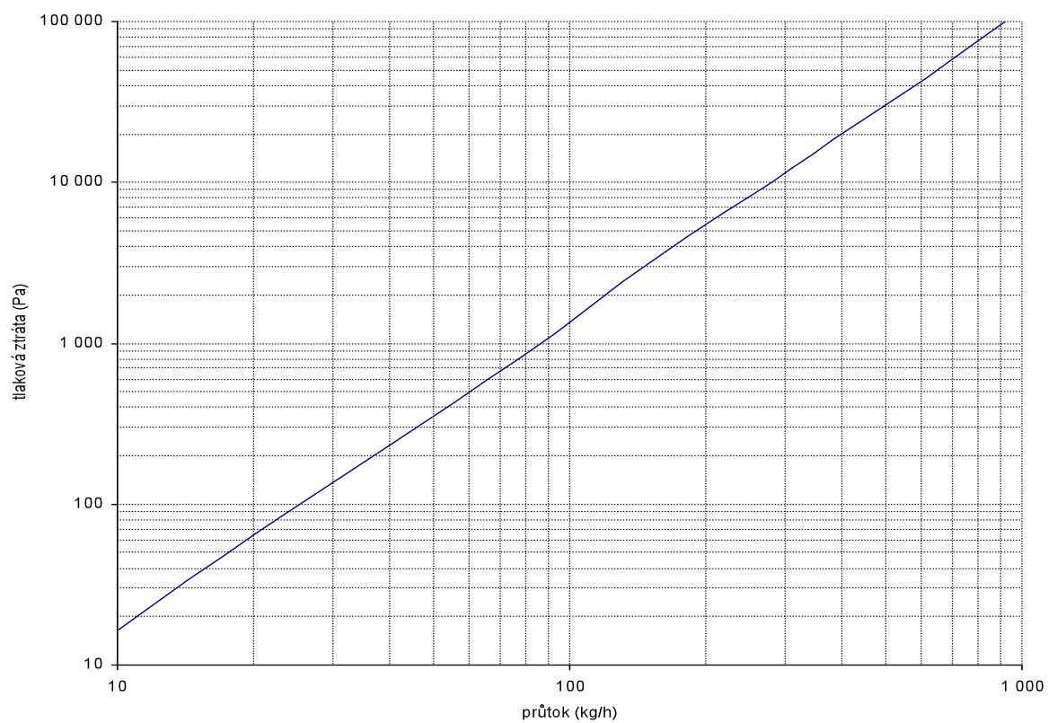
tlaková ztráta ventilového spodku termostatické hlavice 1/2" rohového
